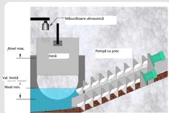
Diagrama schematică a stației de ridicare ape uzate
